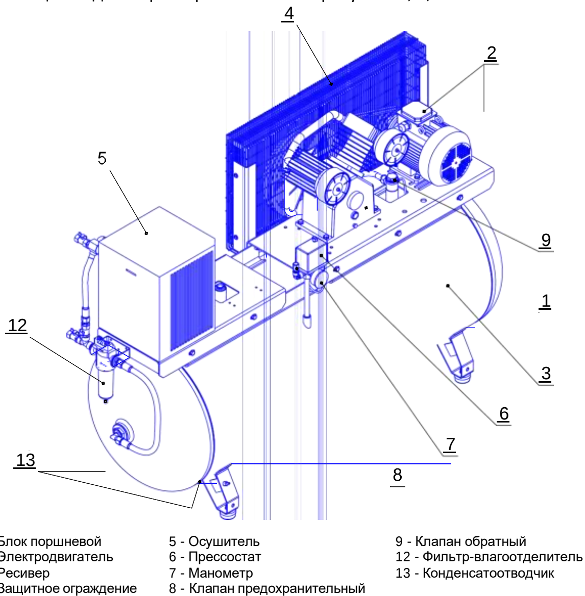
Рисунок 3 - Общий вид компрессора CB4/Φ-500.LB50Д
